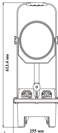
Габаритные размеры светильника [мм]
