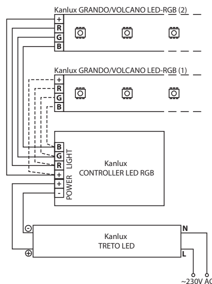
Примерная схема системы питания и управления цветом линейных модулей LED RGB Зразкова схема живлення та керування барвою лінійних модулів LED-RGB
