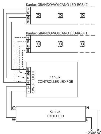
Примерная схема системы питания и управления цветом линейных модулей LED RGB Зразкова схема живлення та керування барвою лнійних модулів LED-RGB
