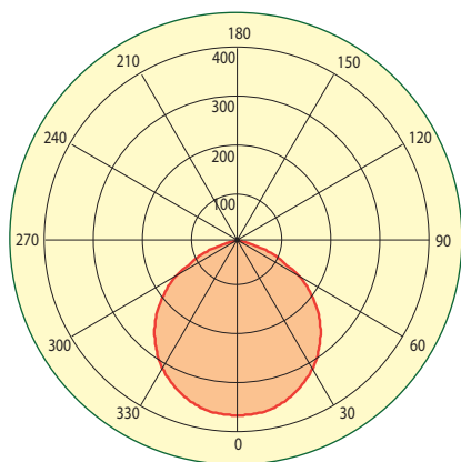
Кривая силы света «Д» (нормализованная диаграмма) ILLUMINATION PHYTO 60
