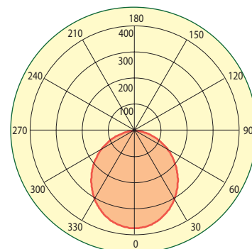
«Д» для артикулов РНУТО 400 и РНУТО 800
