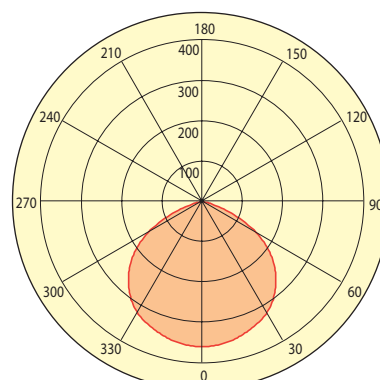
Кривые силы света, кд/1000 лм (нормализованные диаграммы)
