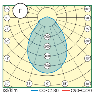
«Д», «Г», «К» для серии INDUSTRY 3
