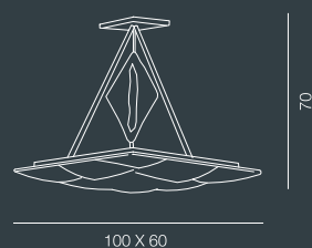
2552/L10L 10 x max 40W G9 230V CE
