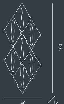
2552/PL7L 7 x max 40W G9 230V CE
