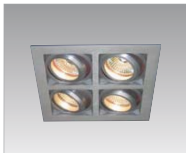
Модель: FE1314 Цвет: AL, G Врезной диаметр: 14,2x14,2 см Лампа: MR16
