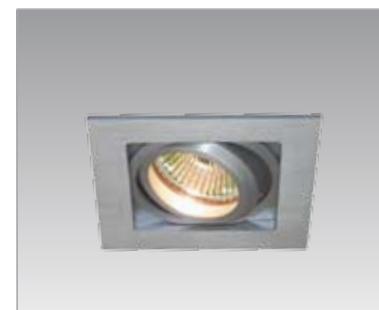
Модель: FE1311 Цвет: AL, G Врезной диаметр: 9,2 см Лампа: MR16
