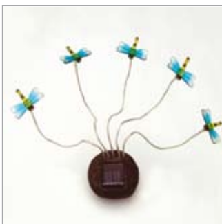
Модель: ST-9002 Светодиод: 5LED Цвет: желтый, голубой, прозрачный
