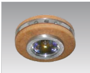
Модель: DN7238 Цвет: AL Цвет: W, Y, Brown Врезной диаметр: 5,7 см Лампа: MR16
