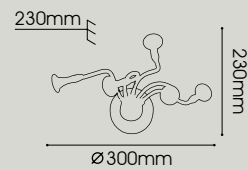
LT06-2228/03.3.5 Gargona G4 MAX 20W x 5
