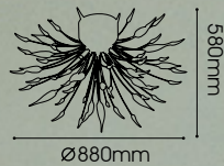
LT06-2252/03.1.16 Chili G4 MAX 20W x 16
