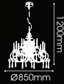
LT06-2213/02.2.15 Constancia G4 MAX 20W x 15
