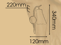
LC05-5450/1W Tiffany E14 MAX 60W x 1
