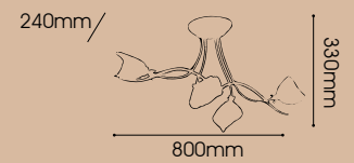
LC05-5446/4C Flower G9 MAX 40W x 4
